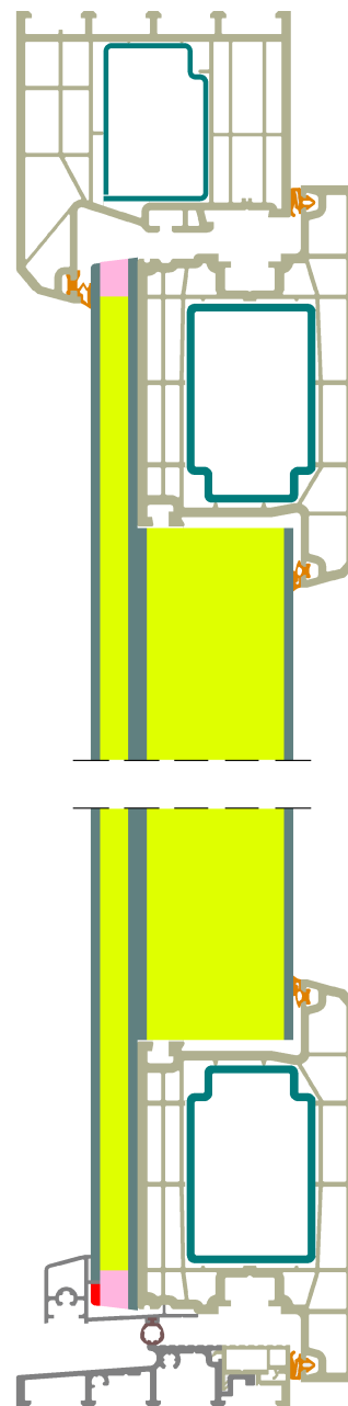
Vertikalschnitt
