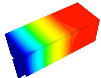
Isothermenbild des Horizontalstabes
