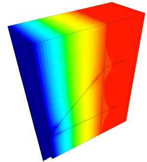
Isothermenbild des Dreiecks
