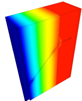
Isothermenbild des Schrägstabes
